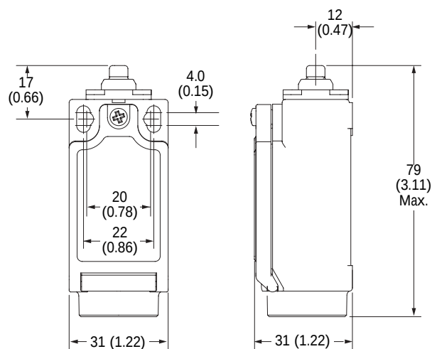
Dome Plunger
