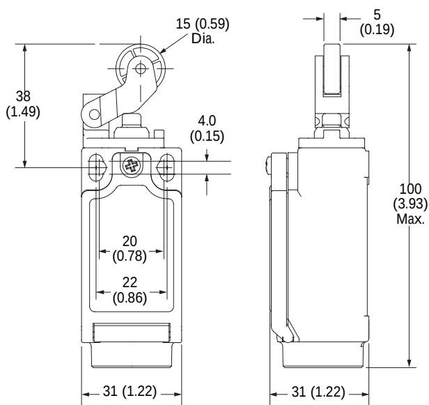
Hinge Lever
